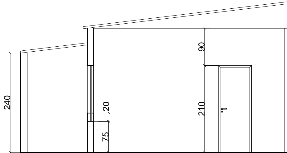
Corte B-B
