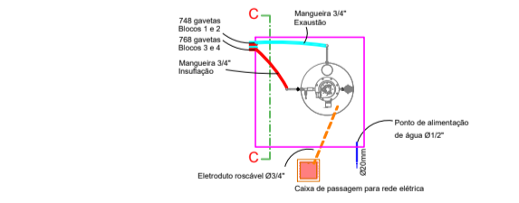
Esquema de ligação da Casa de Máquinas Esc.: 1-100
