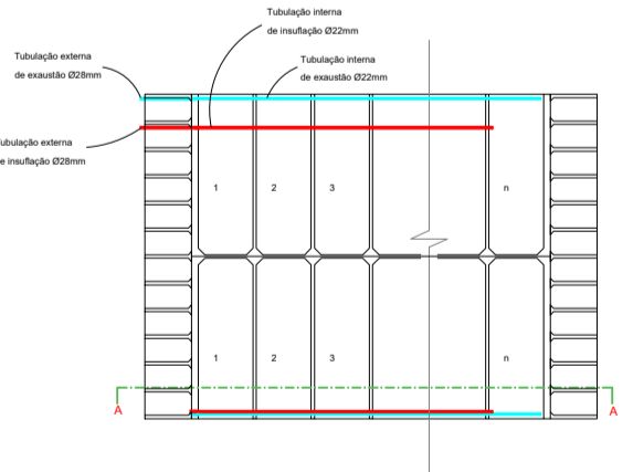
Esquema de ligação das gavetas Esc.: 1-100
