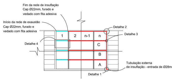
Corte esquemático A-A Esc.: 1-100
